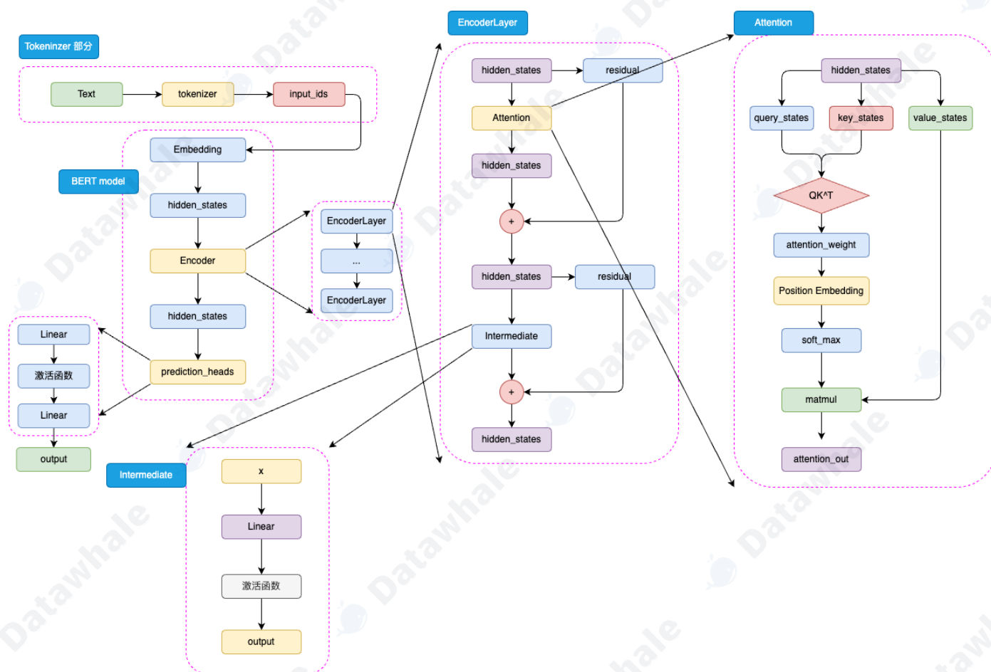
图3.1 BERT 模型结构
